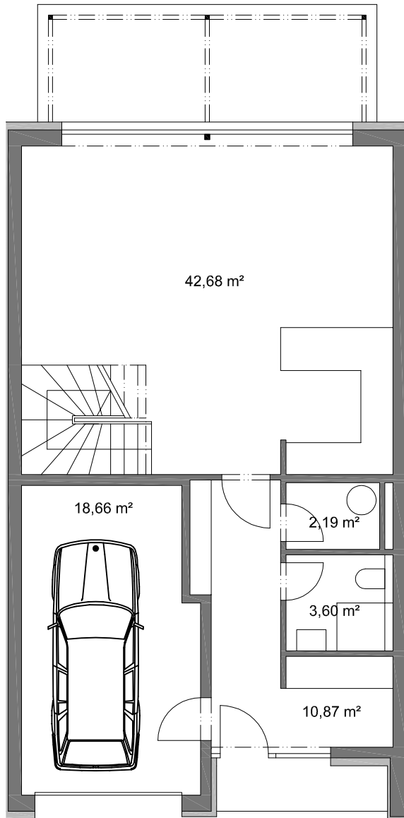
1.NP
