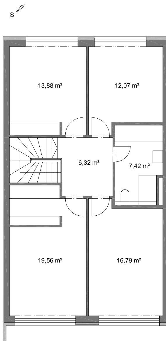
2.NP
