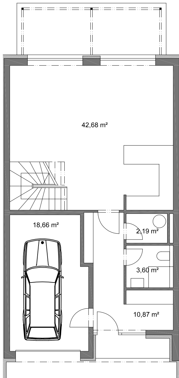
1.NP
