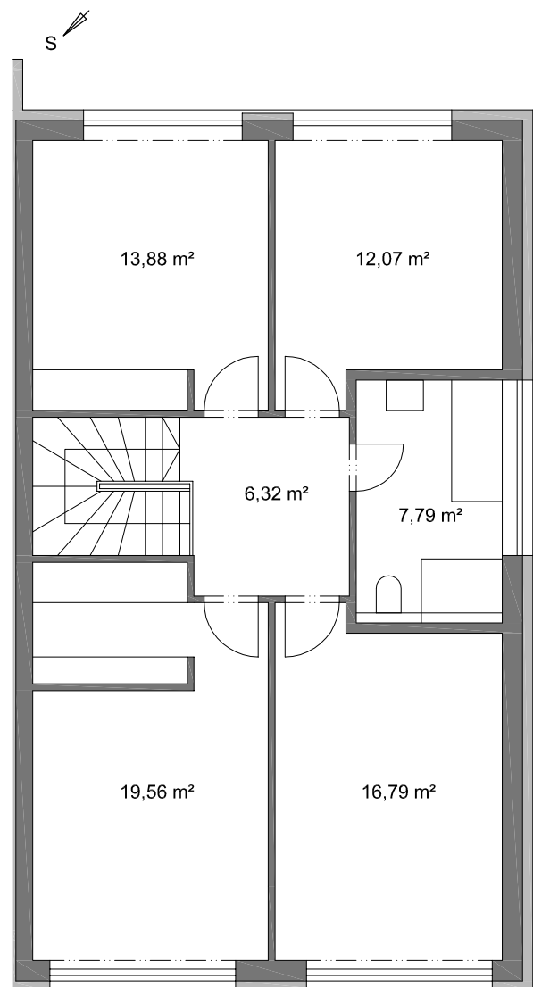
2.NP
