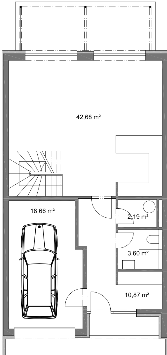
1.NP
